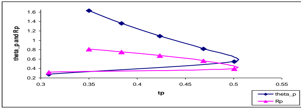
شكل (5) تقديرات المعلمة ودالة المعدلية (p) ( \sum t_p = 2.43518, \delta = 9 )
