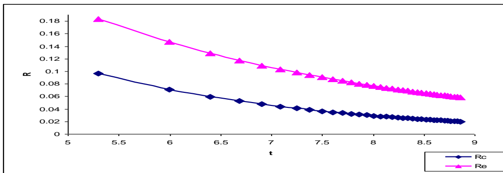
شكل (4) تقديرات دالة المعدلية لمنحنى النمو داينى
