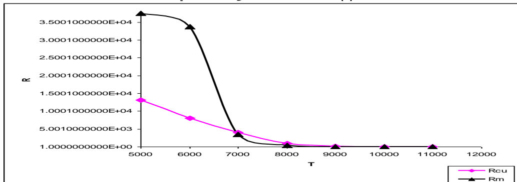
شكل (2) تقديرات دالة المعدلية لمنحنى النمو المثالي
