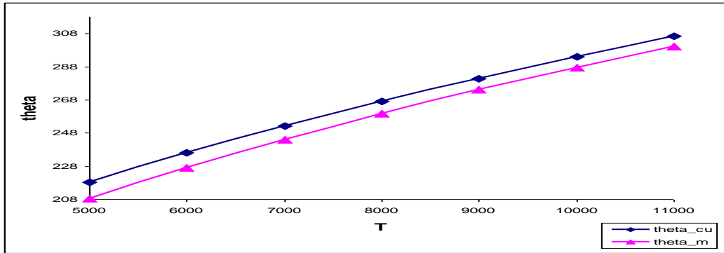
شكل(1) تقديرات معلمات منحنى النمو المثالي
