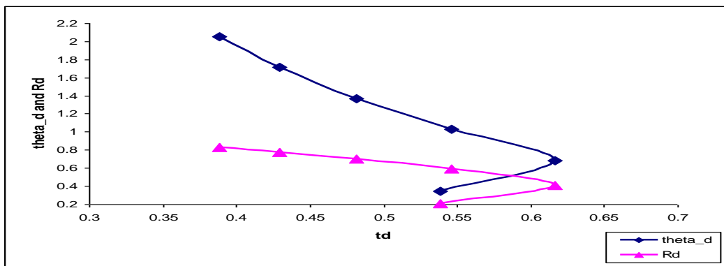
شكل (6) تقديرات المعلمة ودالة المعدلية (d) ( \sum \lambda_d = 7.147, tt = 3 )
